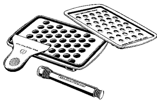
Füllset für 40 Dosierkapseln
